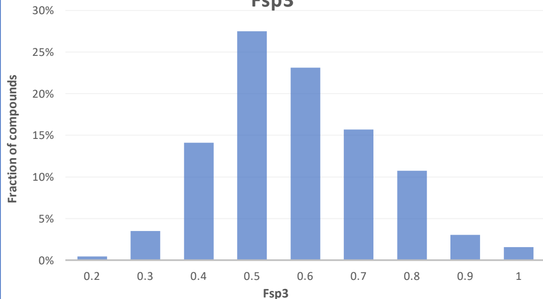
Fsp3
